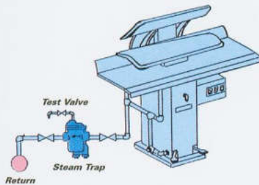
Fig. 4 LAUNDRY PRESS
